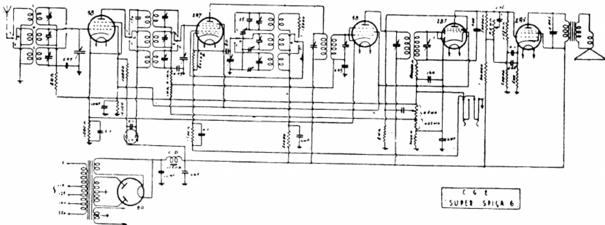
COMPAGNIA GENERALE DI ELETTRICITÀ. — Modelli: « Super Spica 6 trionda, consoltrionda e fonotrionda » Produzione 1935. • Media frequenza: 460 kc.
